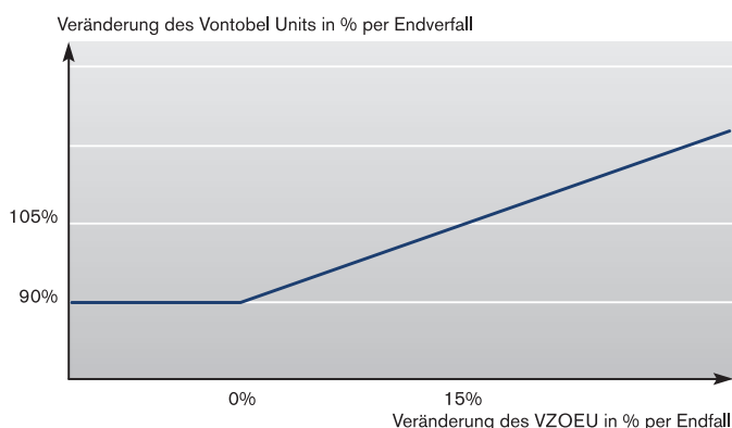
Payoff-Diagramm VUOEU
